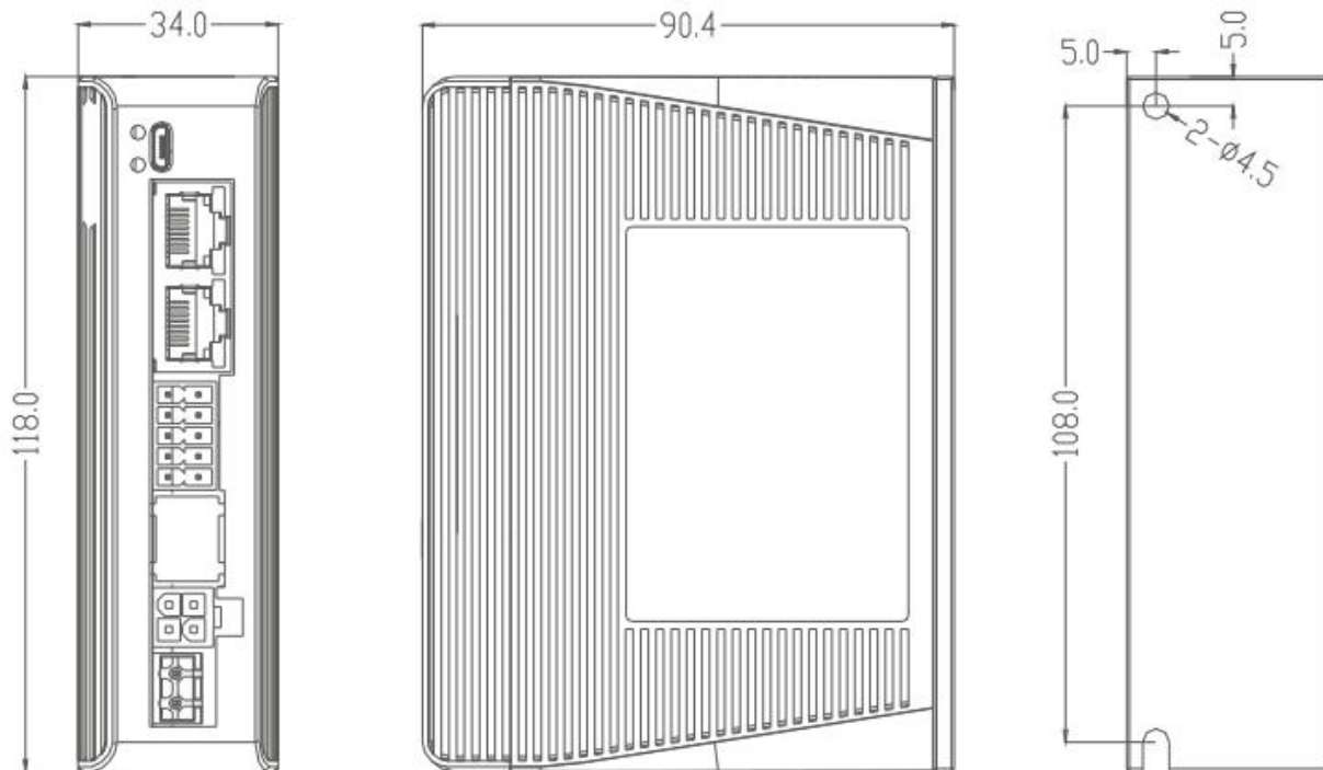
图 2-1 CL3C-EC503/507 安装尺寸图(单位: mm)
