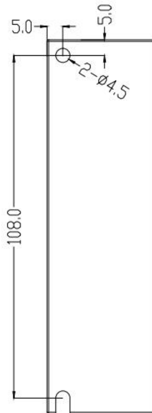
图 2-1 CL3C-EC503/CL3C-EC507 安装尺寸图(单位: mm)
